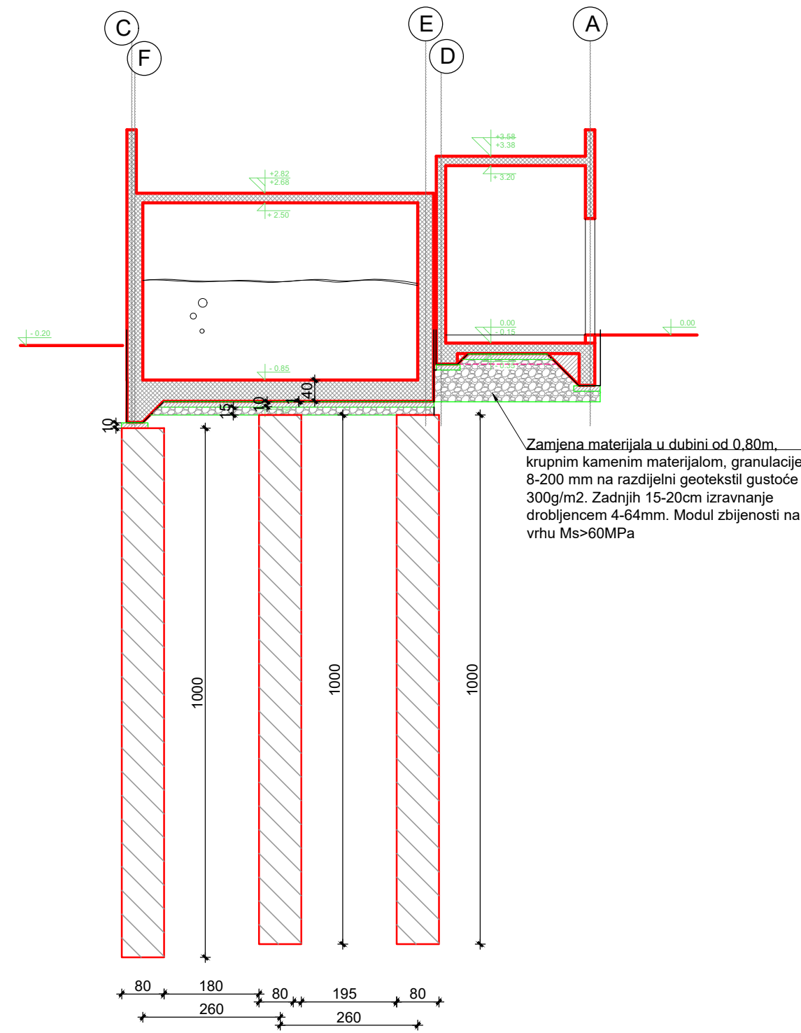
Presjek 2-2 M 1:100
