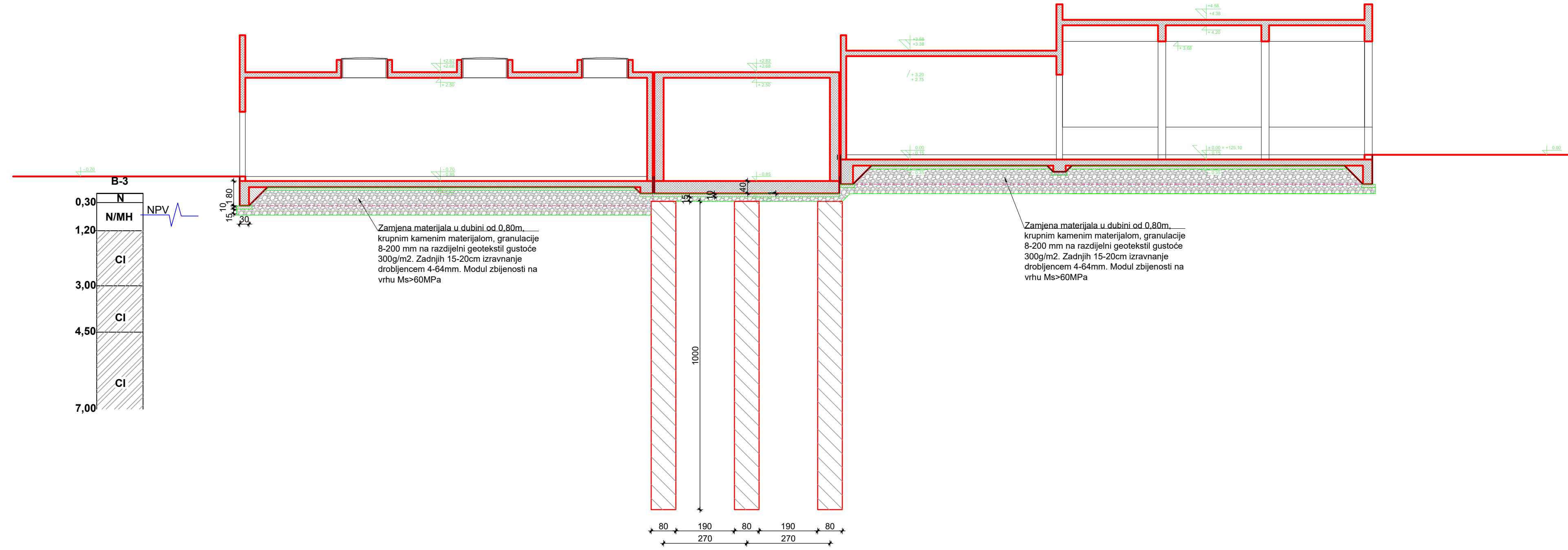
Presjek 1-1 M 1:100
