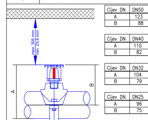
Detalj 2 SPRINKLER MLAZNICA STOJEĆA
